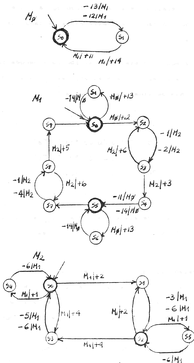
Figura 1 Especificación Convertidor Protocolo de Comunicación
